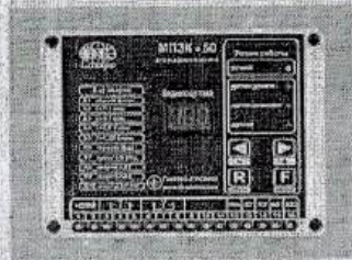
Мікропроцесорний прилад захисту та контролю трифазного електродвигуна МПЗК-50, 150 (5-20А) КАСКАД
